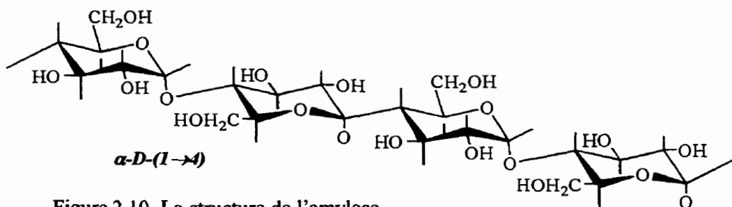
Figure 2.10. La structure de l'amylose
