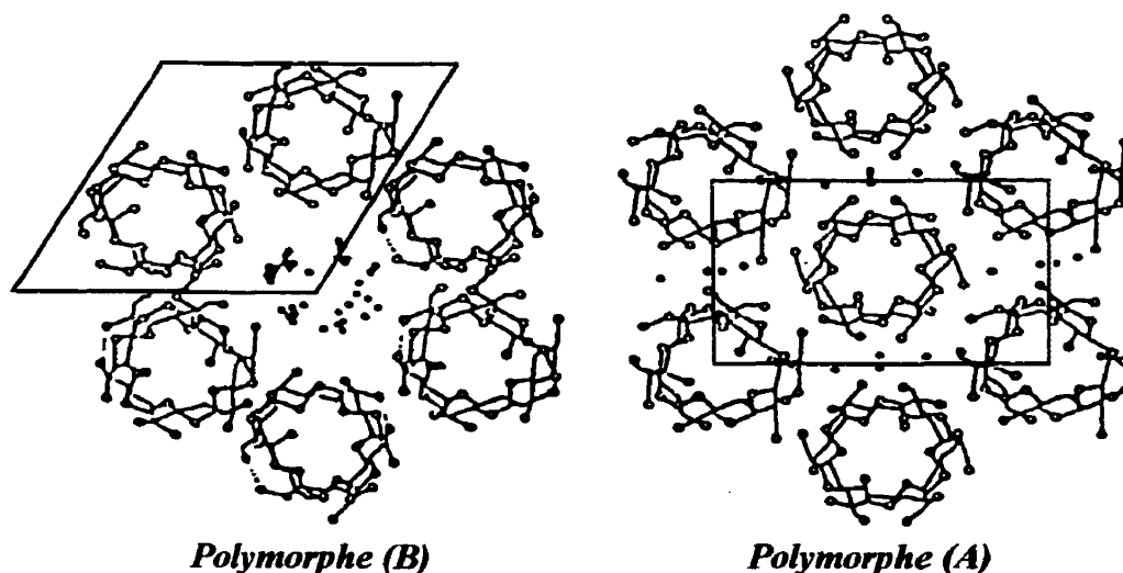
Figure 2.13. Arrangement hexagonal des doubles hélices des chaînes d'amylose: polymorphes (A) et (B) (Wu and Sarko, 1978a)
