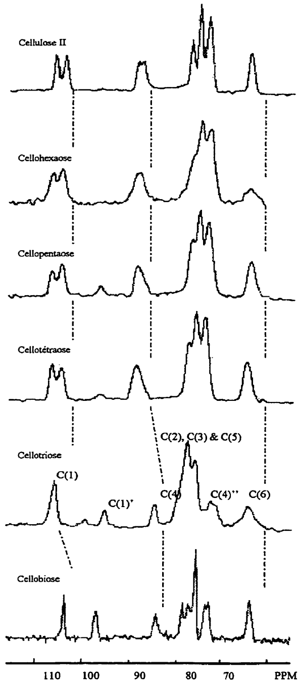
Figure 2.6. Spectres ^{13}\text{C} RMN CP/MAS des oligomères cellulosiques (Dudley et al., 1983)
