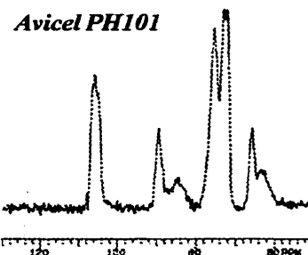
Figure 6.2. Spectres ^{13}\text{C} RMN CP/MAS de l'Avicel PH101® et la CLC-C25
