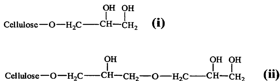
Figure 2.8. Représentation schématique des produits secondaires de la réaction de l'épichlorhydrine avec la cellulose: (i) cellulose glycéryle monoéther, (ii) cellulose glycéryle monoéther secondaire
