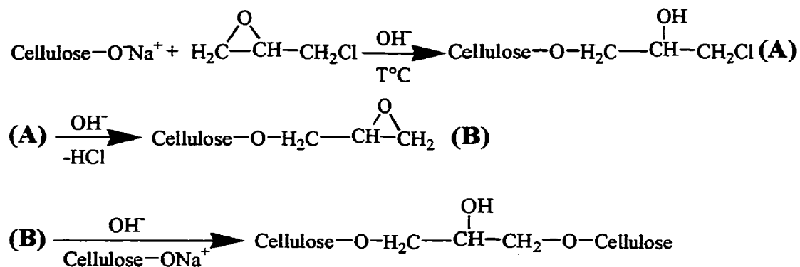
Figure 2.7. Représentation schématique de la réticulation de la cellulose par l'épichlorhydrine (McKelvey et al., 1963)
