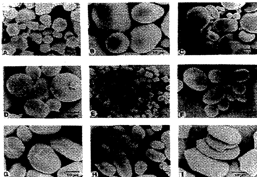
Figure 2.9. Photographies des granules d'amidon obtenues par microscopie électronique à balayage: A) Maïs, B) Pomme de terre, C) Blé, D) Seigle, E) Riz, F) Fève, G) Pois, H) Avocatier et I) Shoti. (Jane et al., 1994).
