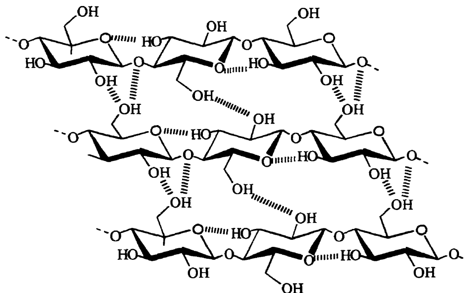
Figure 2.3. Ponts hydrogène intermoléculaires entre les chaînes cellulosiques
