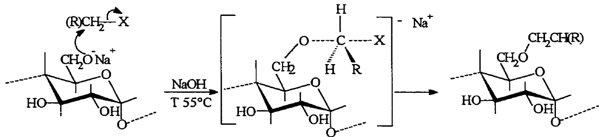
Figure 6.4. Représentation de la synthèse d'un polymère SA à partir d'un substituant halogénure.
