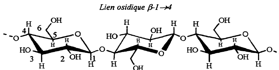
Figure 2.2. La structure de la cellulose
