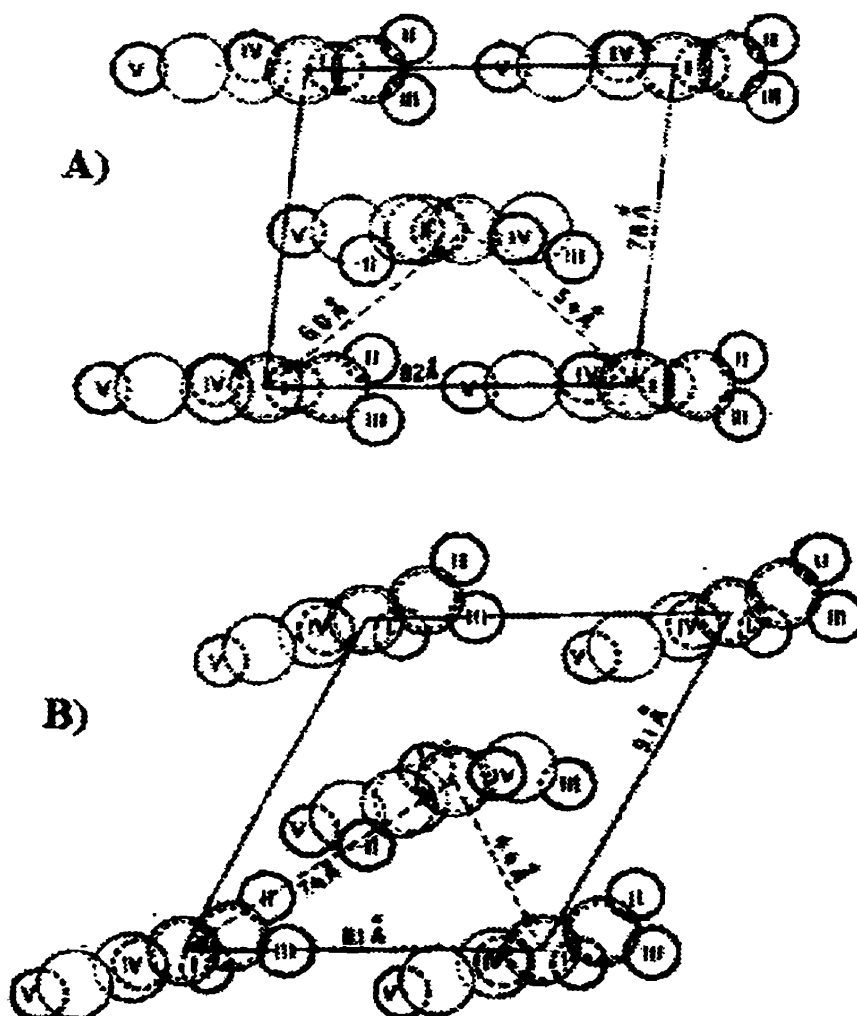
Figure 2.5. Projection de la maille élémentaire de la cellulose. A) Cellulose native (I) et B) Cellulose mercerisée (II) (Champetier, 1933; Encyclopedia of Polymer Science and Engineering, 1985a)
